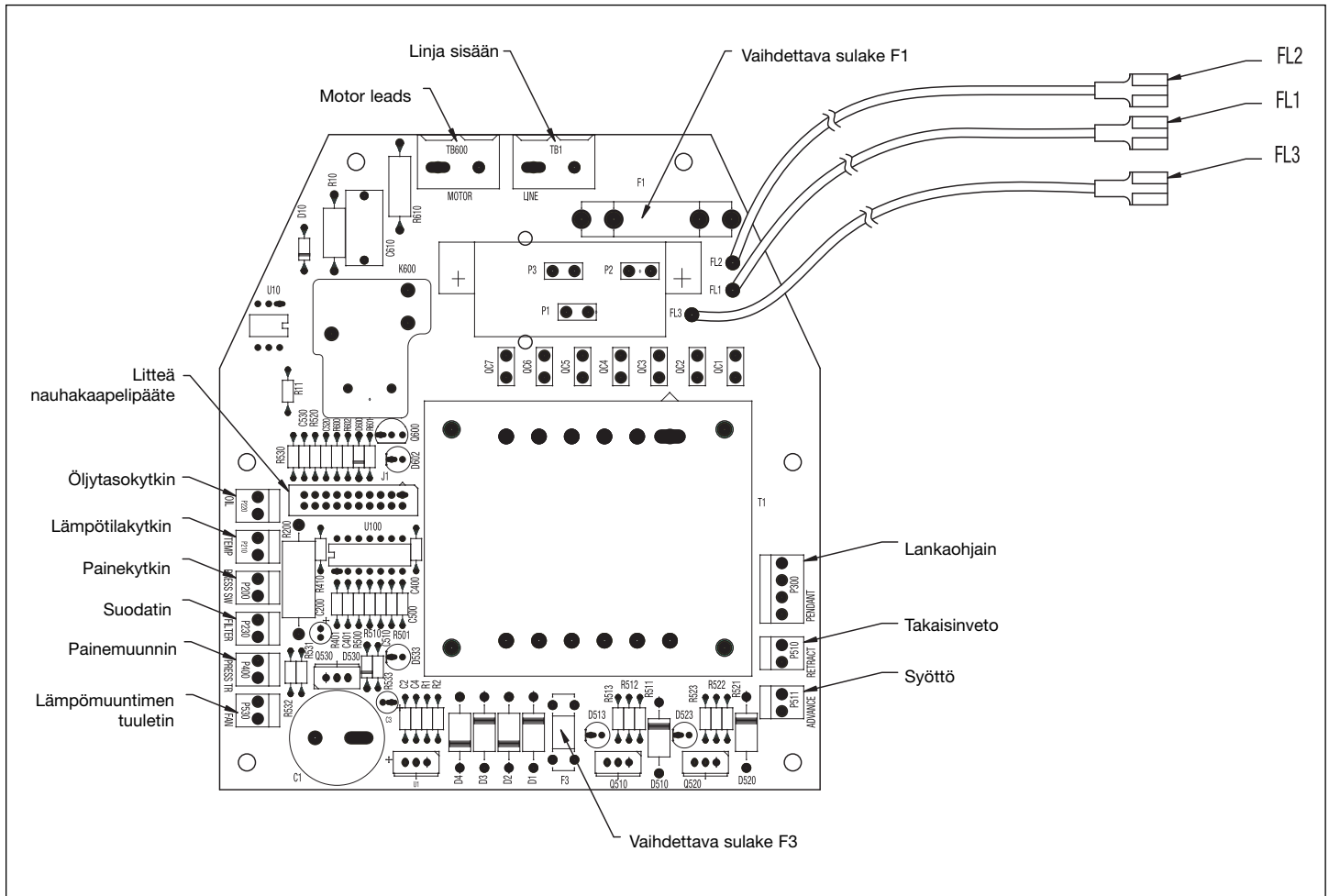
Kuva 11, sähkövirtapaneelin kokoonpano
