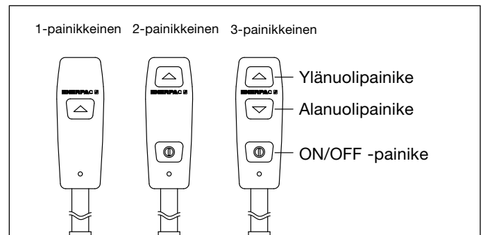
Kuva 8, lankaohjaimen painikevaihtoehdot
