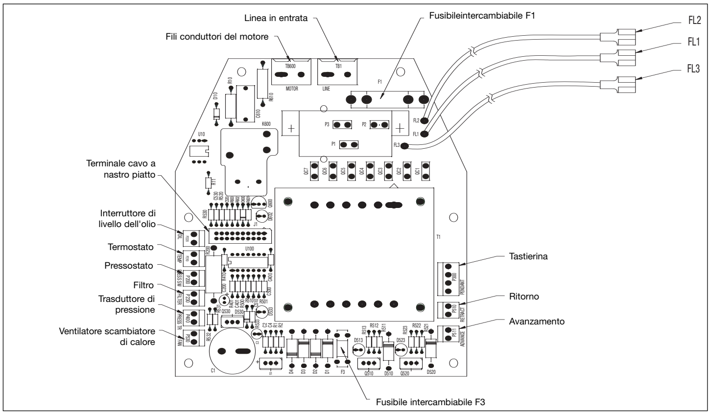
Fig. 12, Configurazione pannello alimentazione elettrica
