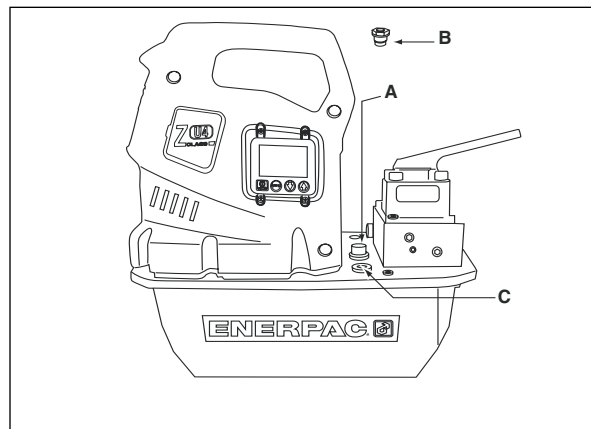
Figuur 2, installatie ZU4 ontluichter
