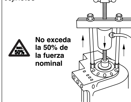
ilustración 3 - Empuje con un extractor de cojinetes
