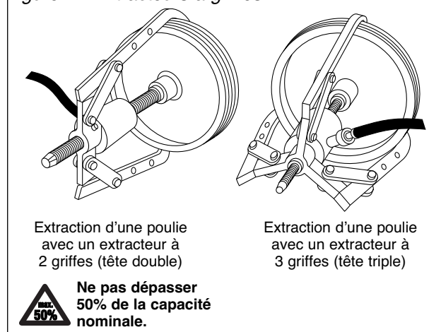
figure 1 - Extracteurs à griffes
