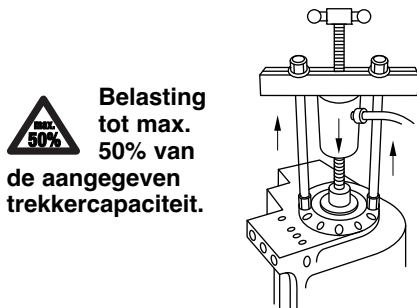
illustratie 3 - Oppersen met 2-armig brugstuk
