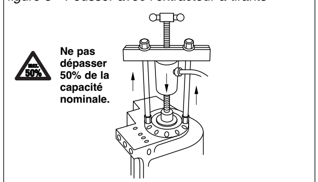
figure 3 - Pousser avec l'extracteur à tirants
