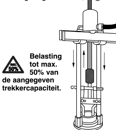
illustratie 2 - toepassing van brugstuk met inwendige lagertrekker
