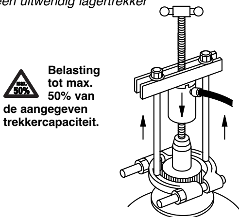
illustratie 4 - 2-armig brugstuk in combinatie met een uitwendig lagertrekker
