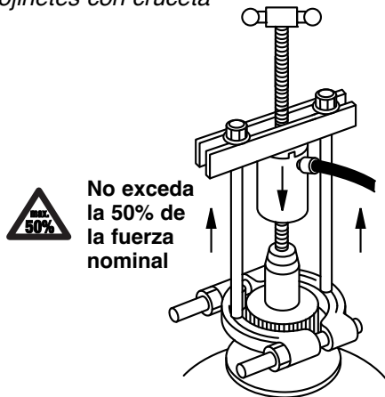
ilustración 4 - Accesorio para extracción de cojinetes con cruceta
