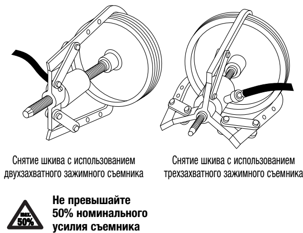
Рис. 1. Зажимные съемники
