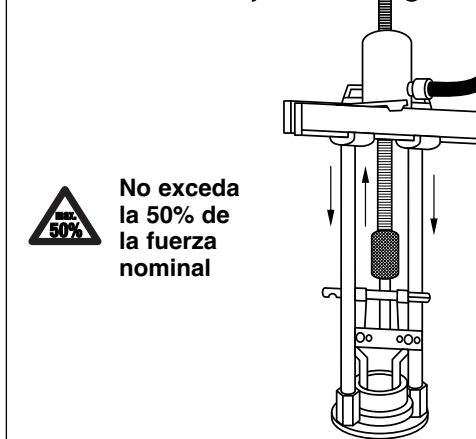
ilustración 2 - Cruceta con accesorio de extracción de cubos de cojinete
