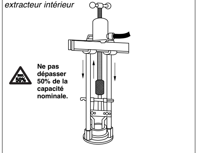
figure 2 - Tête d'extracteur avec accessoire extracteur intérieur
