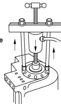
Abbildung 3 - Pressen mit dem Jochabzieher
