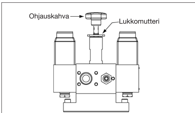
Kuva 7, varoventtiili
